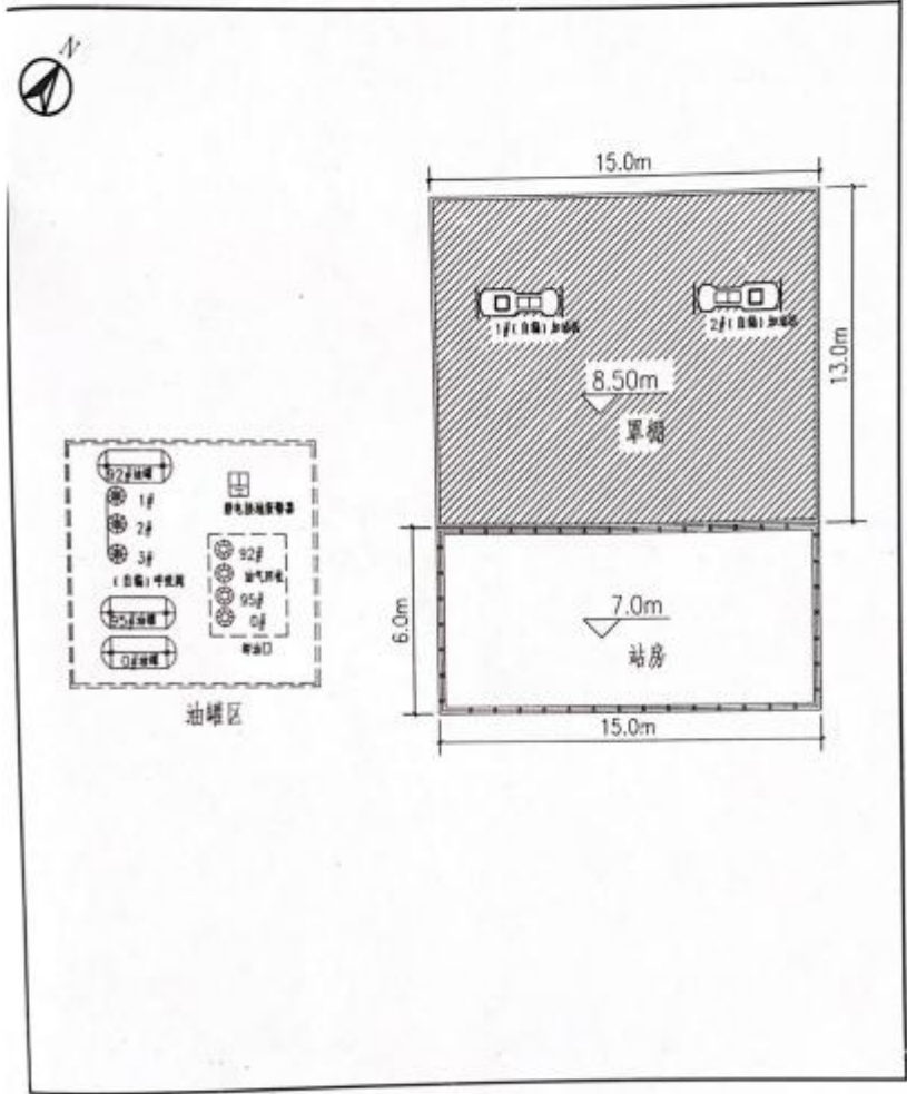
接闪器布置及保护范围图
